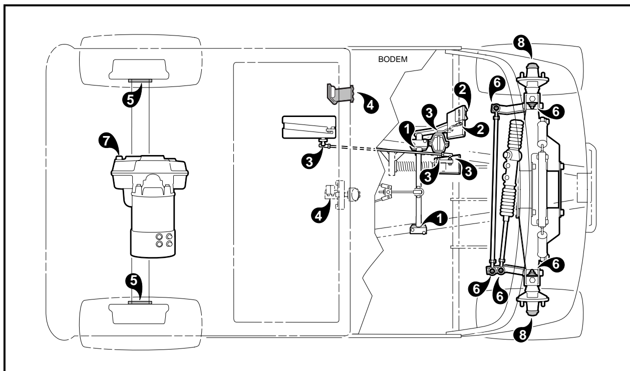
Figuur 11 Smeerpunten van het voertuig
