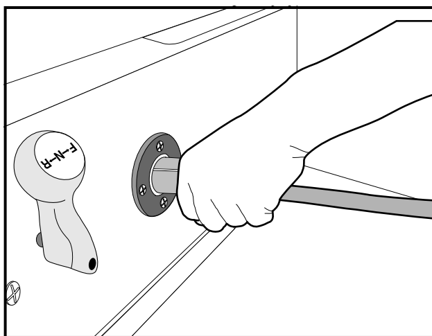
Figuur 13 Juist insteken van de gelijkstroomstekker van de lader
