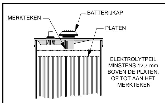
Figuur 12 Elektrolytpeil in batterijen
