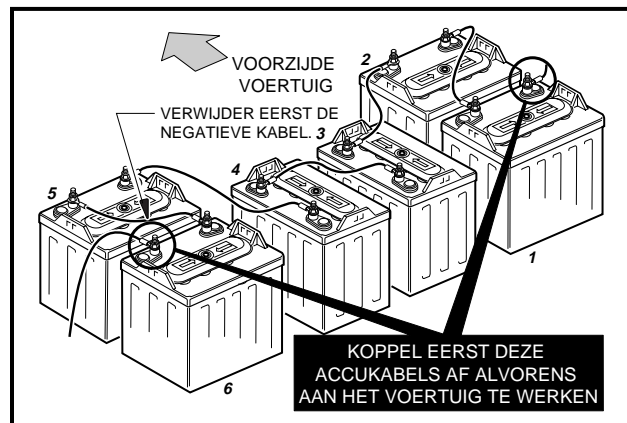
Figuur 2 PowerDrive System 48 en PowerDrive Plus voertuigen
